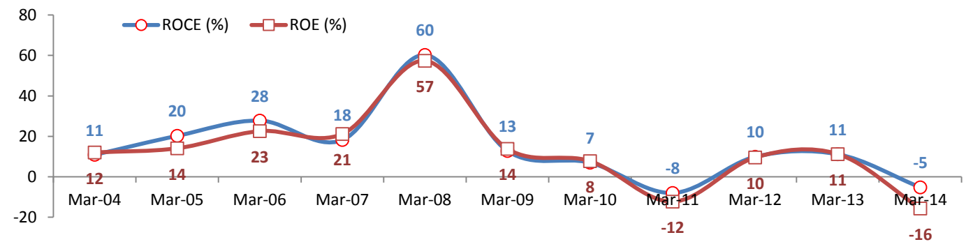
ROCE (%) & ROE (%)
