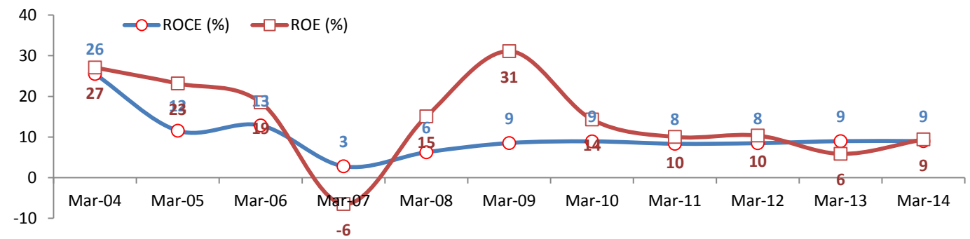
ROCE (%) & ROE (%)
